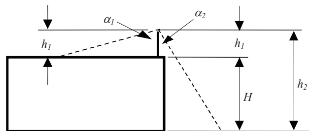
Fig. 6.8 – Volum protejat printr-o tijă de captare verticală
