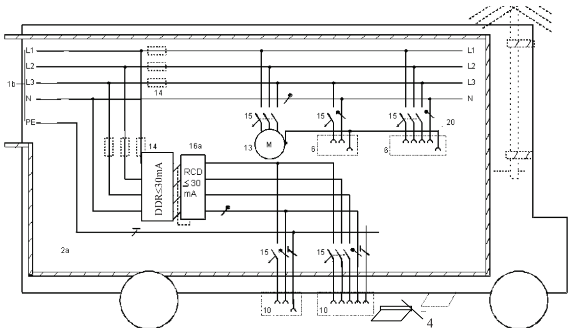
Figura 7.13.4 – Același exemplu cu protecție prin legătură de echipotenzializare locală nelegată la pământ cu o carcasă neconductoare în interiorul unității
