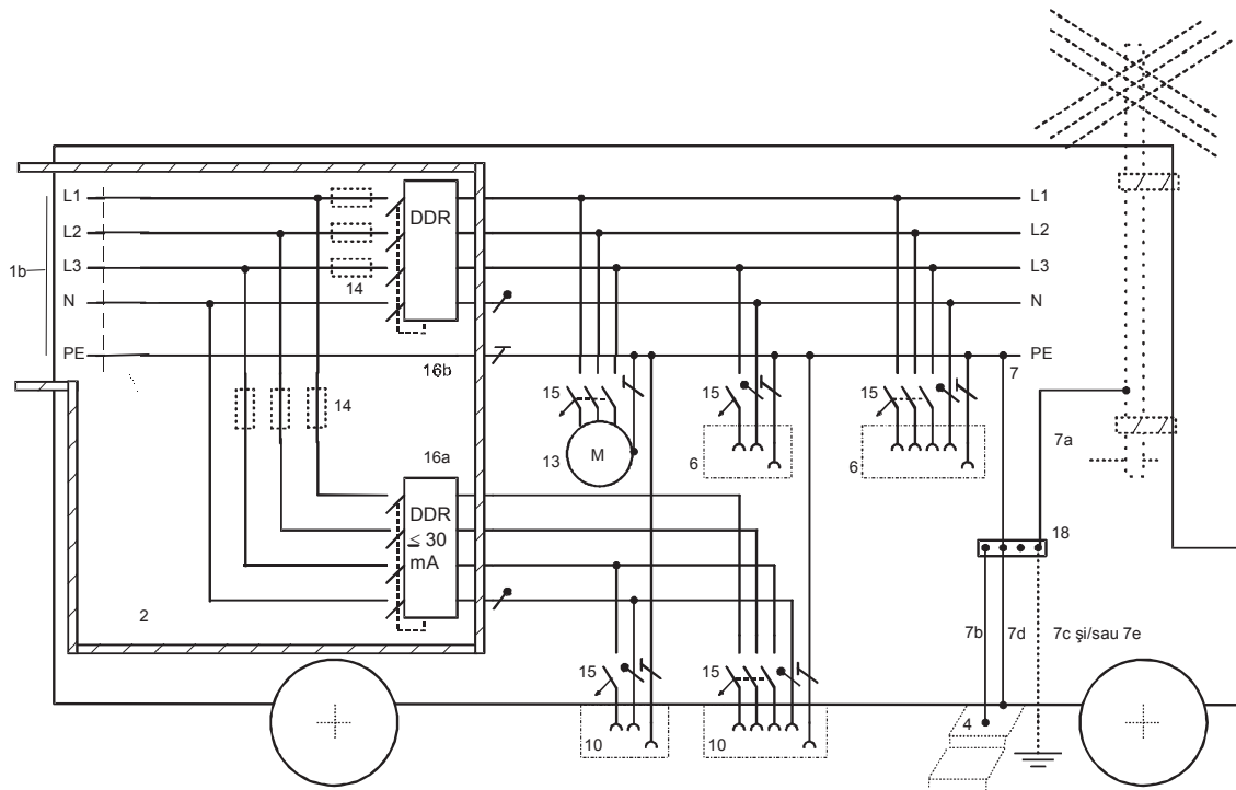
Figura 7.13.3 – Exemplu de conectare la toate tipurile de rețele legate la pământ a unei instalații fixe cu întreruperea automată a alimentării prin dispozitive de curent diferentțial rezidual (DDR), cu sau fără priză de pământ
