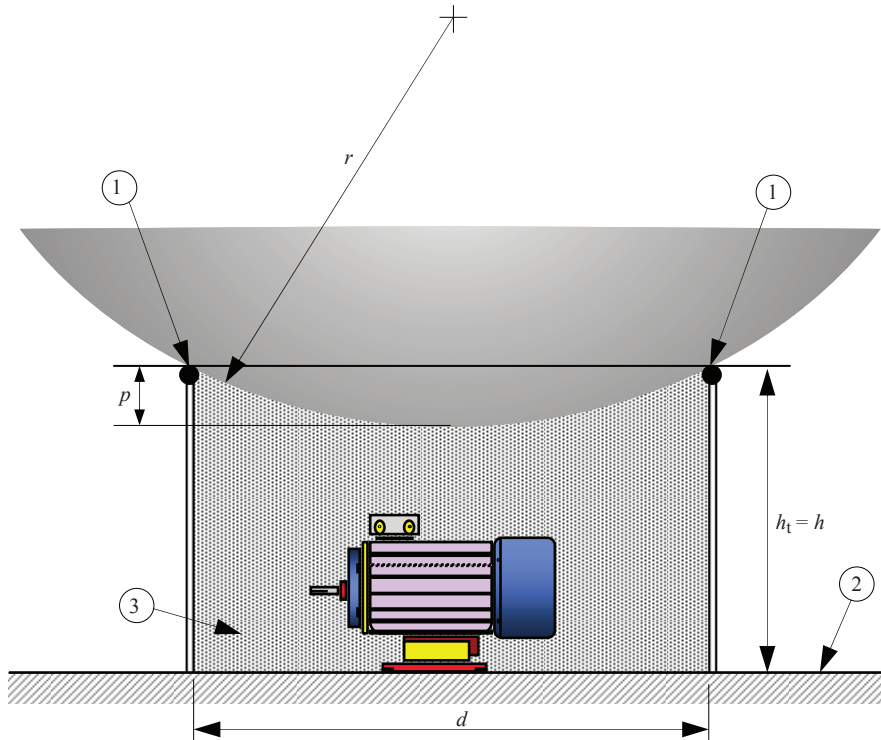
Fig. 6.15 – Volum protejat de două conductoare întinse paralele și orizontale sau de două tije de captare ( r > h_t )
